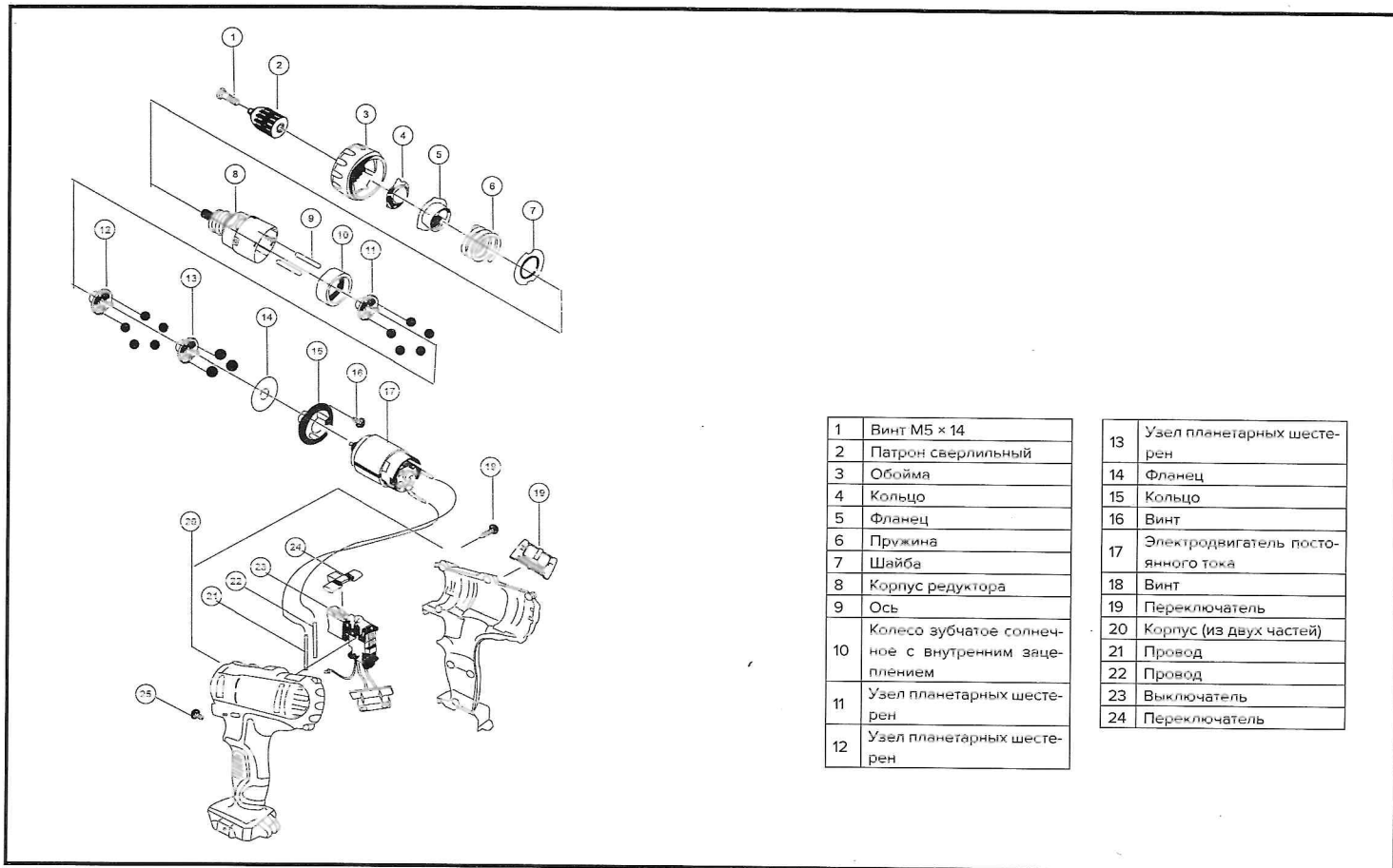
Дрель-шуруповерт аккумуляторная CDB-12-Li-1,5; CDB-14,4-Li-1,5; CDB-18-Li-1,5 артикул 3 11 01 058, 3 11 01 059, 3 11 01 060
